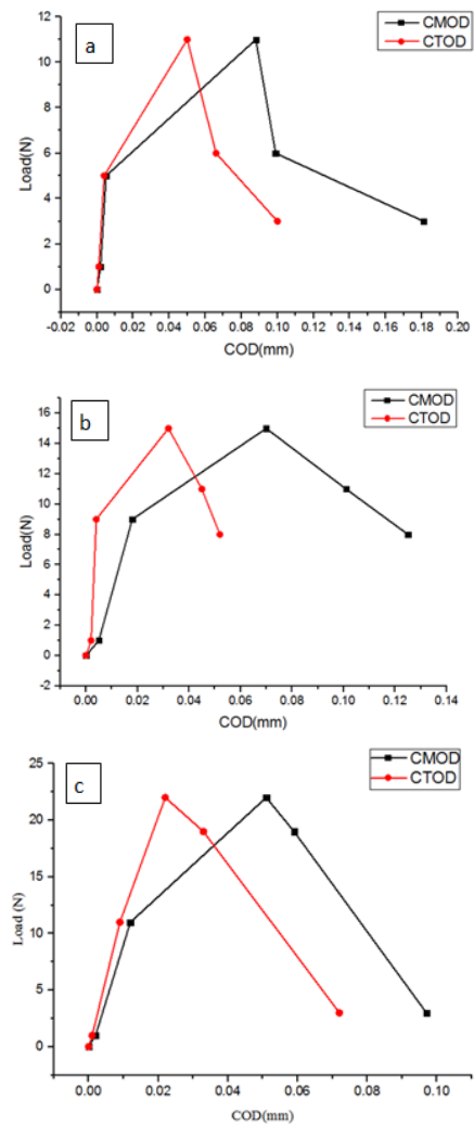
Figure 12. Load versus COD (a) BGC pure, (b) BGC-3wt.% ZrO 2 , (c) BGC-5wt.% ZrO 2
